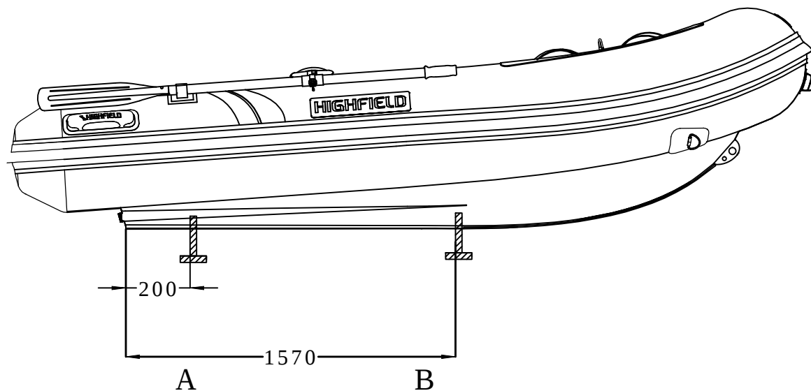
LONGITUDINAL PROFILE
