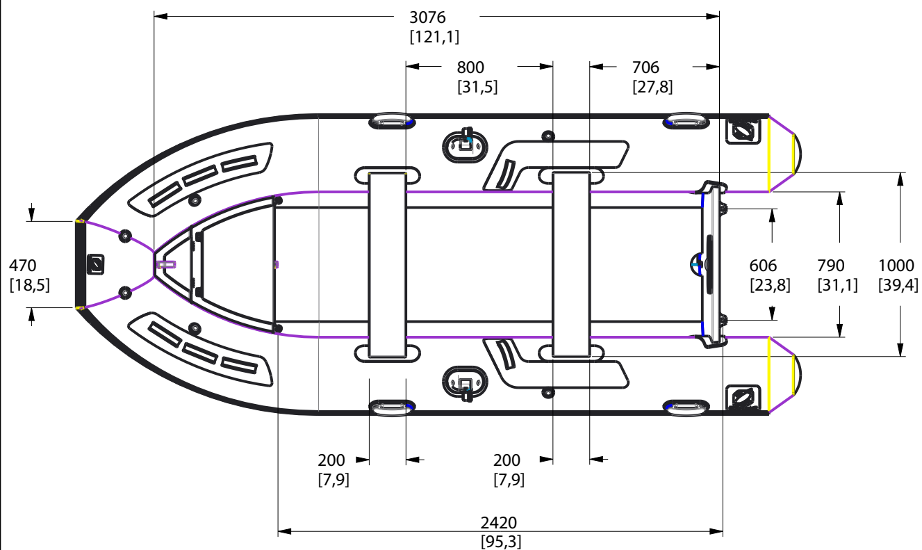
ECHELLE 1:20
