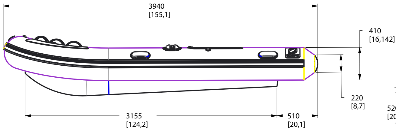
ECHELLE 1:20
