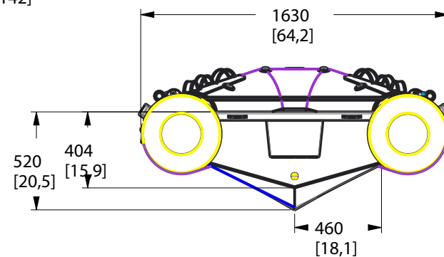
ECHELLE 1:20
