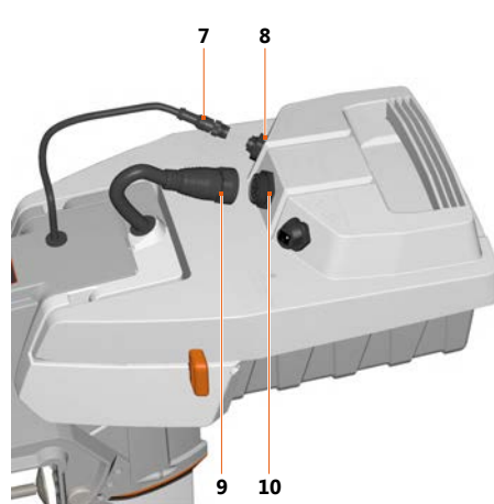
Abb. 11: Elektrische Verbindungen
