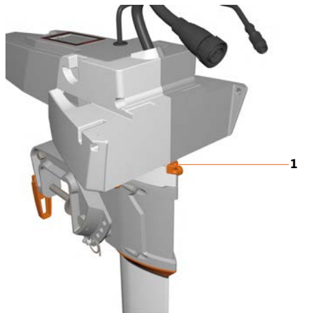
Abb. 12: Position Arretierbolzen
