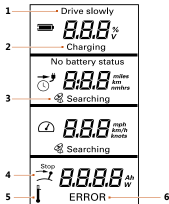
Abb. 17: Multifunktionsanzeige Setup-Menü
