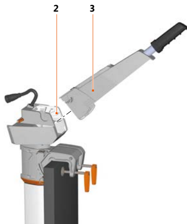
Abb. 8: Montage Pinne
