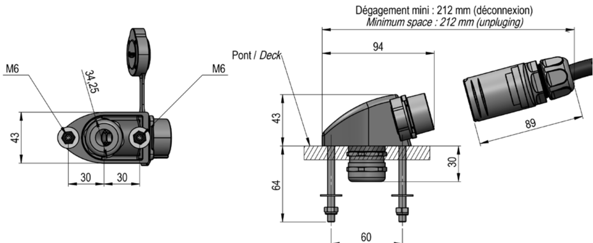
Dimensions prise électrique NEX e LITE 6.5 / NEX e lite 6.5 socket dimensions
