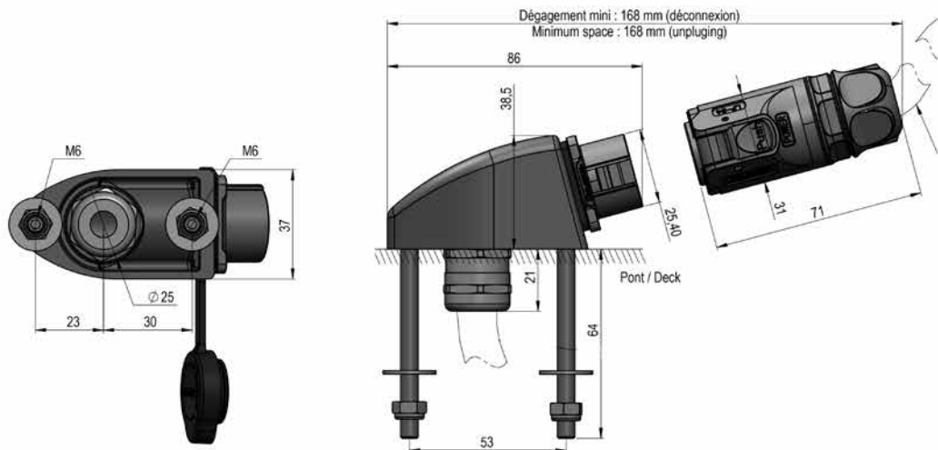
Dimensions prise électrique NEX e LITE 6.5 / NEX e lite 6.5 socket dimensions
