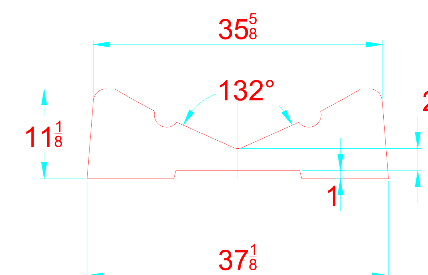
TRANSVERSAL SECTION "B" SECCION TRANSVERSAL "B"
