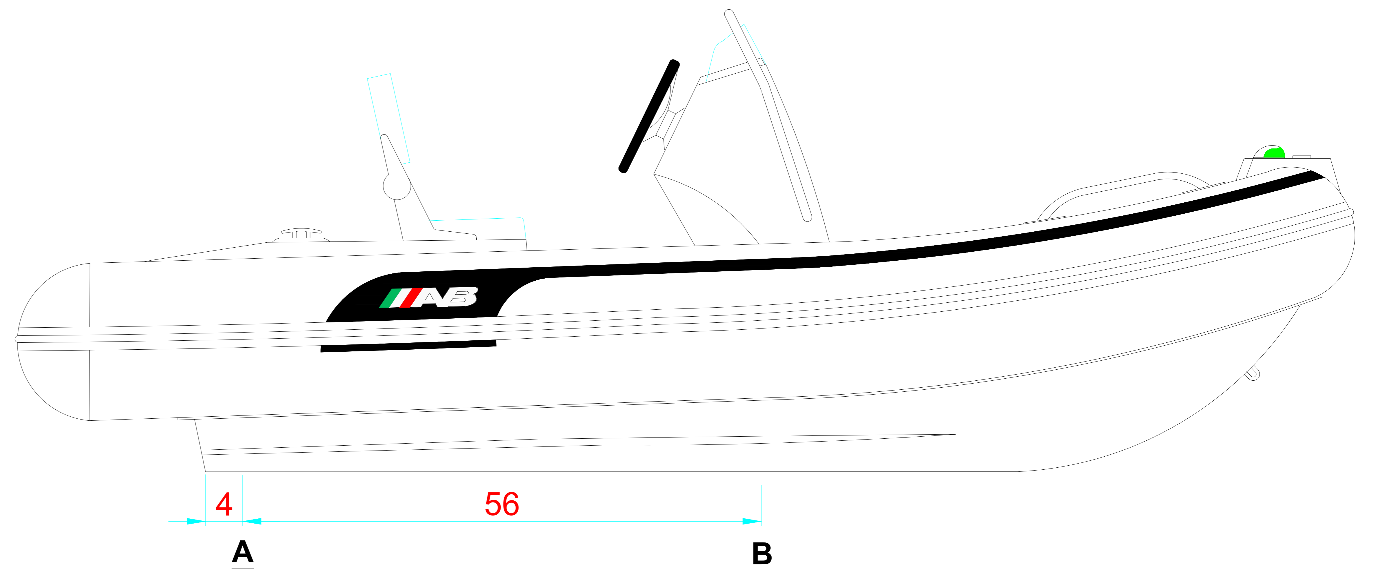
LONGITUDINAL PROFILE VISTA LATERAL
