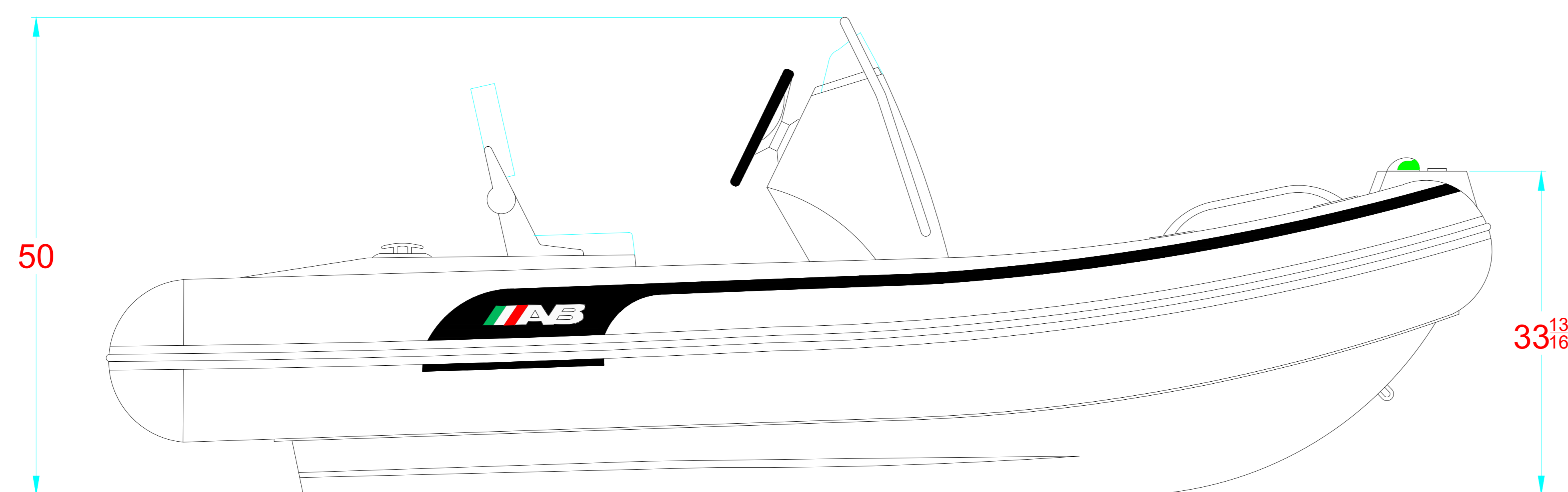
LONGITUDINAL PROFILE VISTA LATERAL
