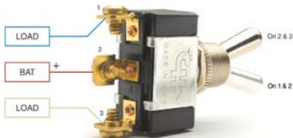
SPDT On-On
